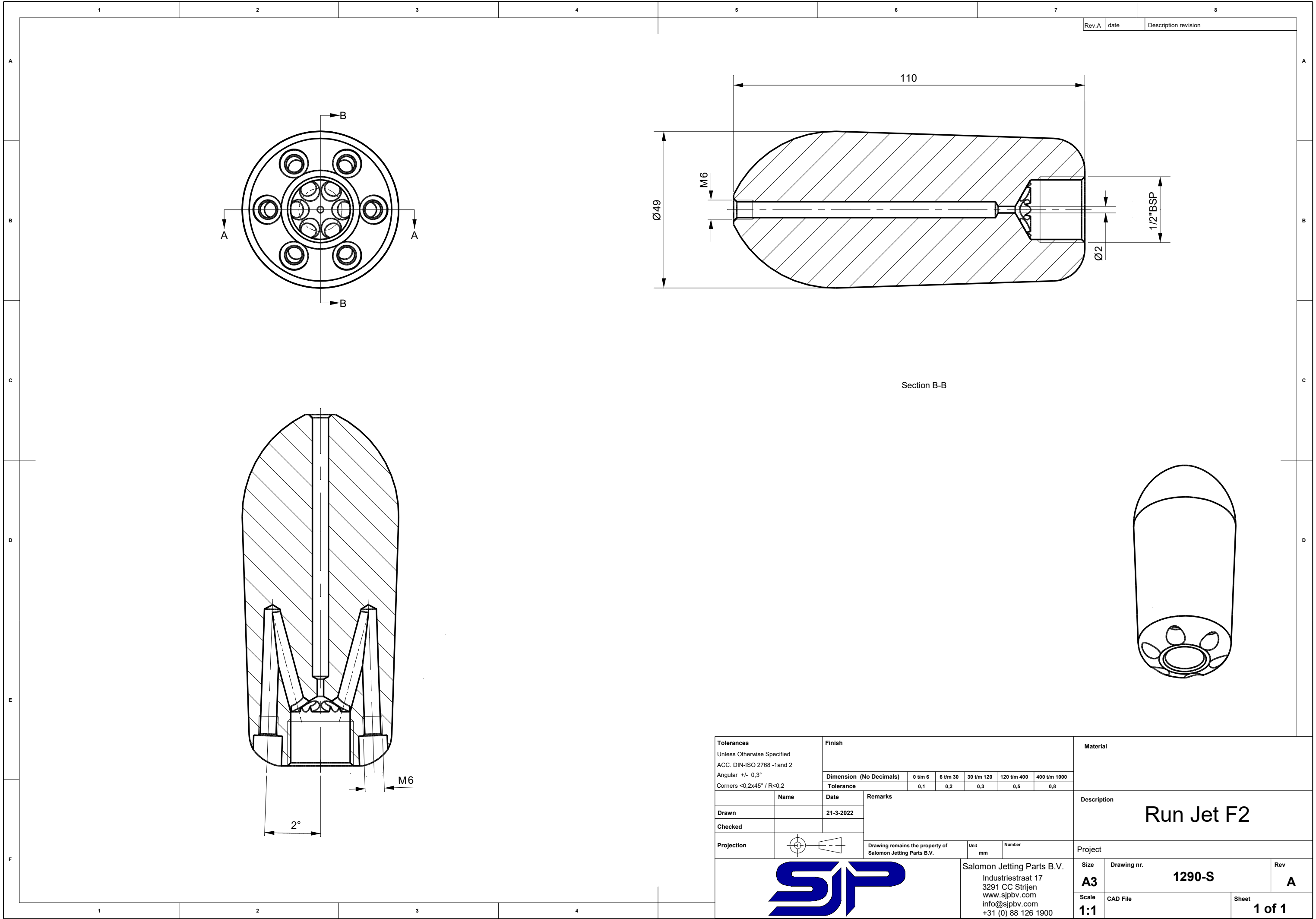
Section A-A
